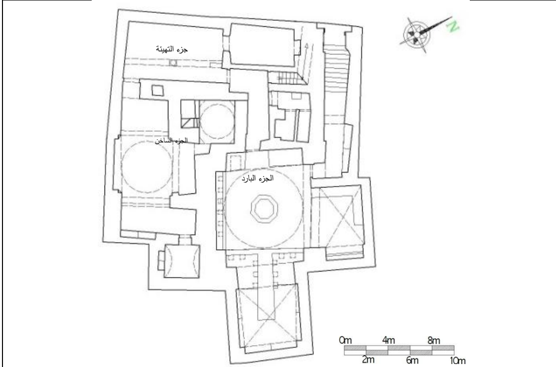
مخطط أفقي يوضح الفراغات المكونة للحمام
